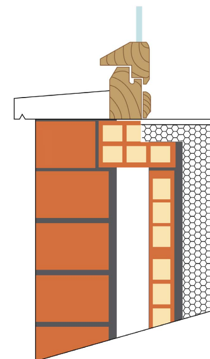
Fig. 27. Detalle 2. Aislamiento térmico por el interior. Encuentro de fachada con alféizar.
