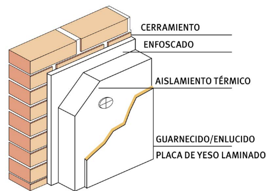
Fig. 9. Esquema del trasdoso con placa de yeso laminado
