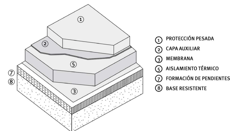
Fig. 11. Esquema de la cubierta invertida
