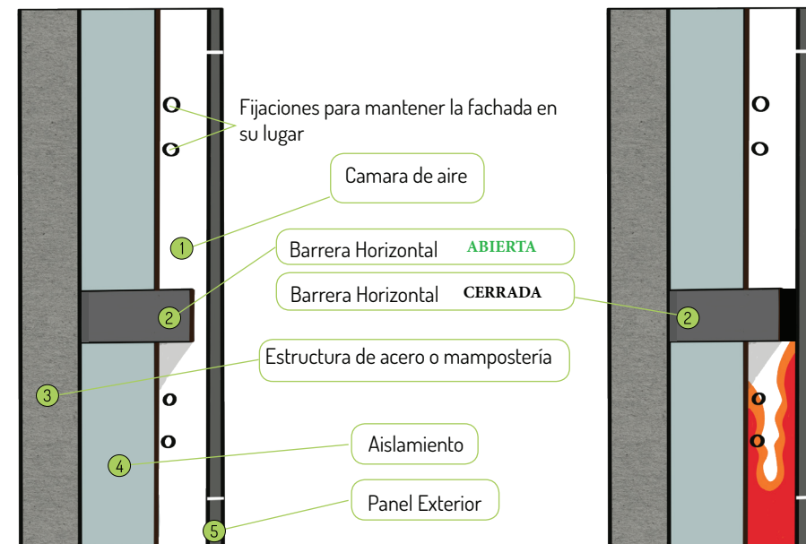
Figura 2. Ejemplo de Fachada Ventilada con barreras
