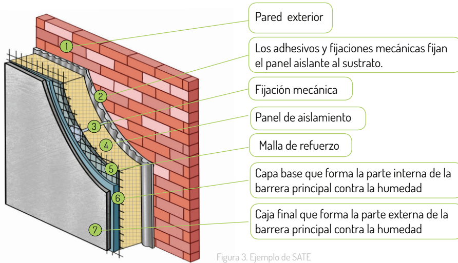
Figura 3. Ejemplo de SATE
